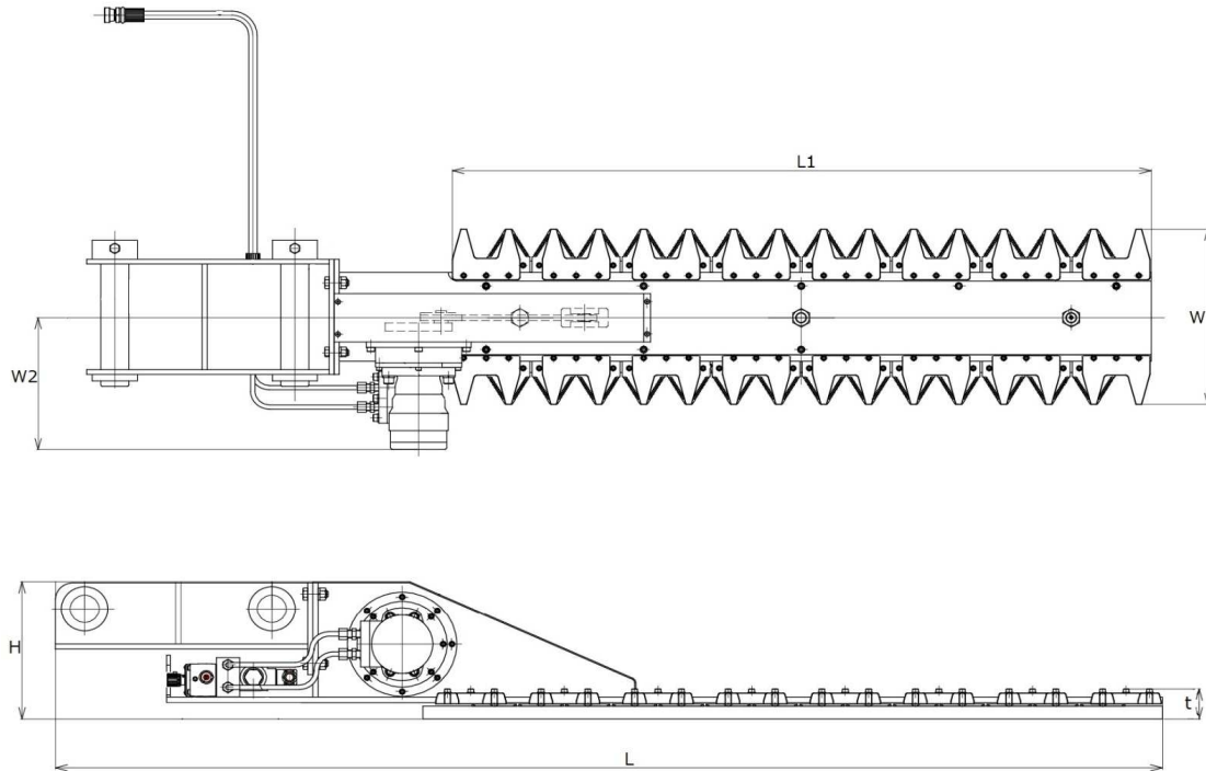
【仕様図】
